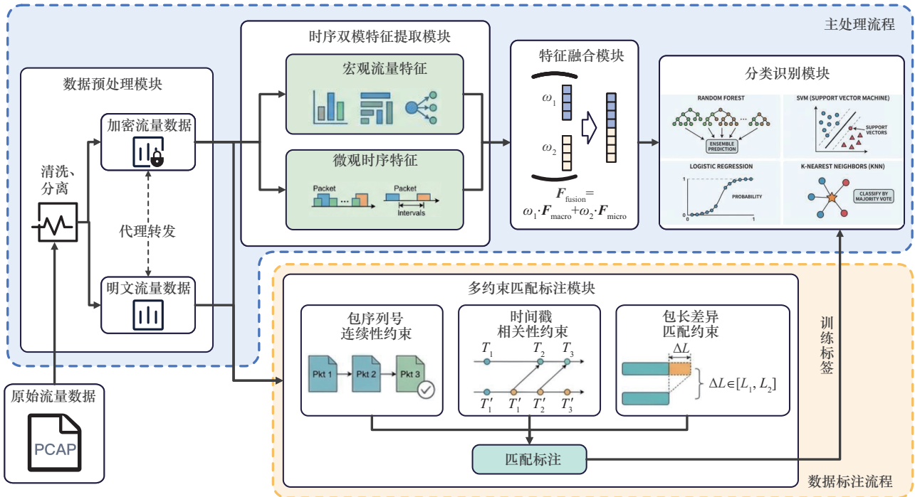
图3 时序双模特征融合框架
